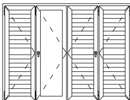
ESQUEMA 422 SCHEME 422
